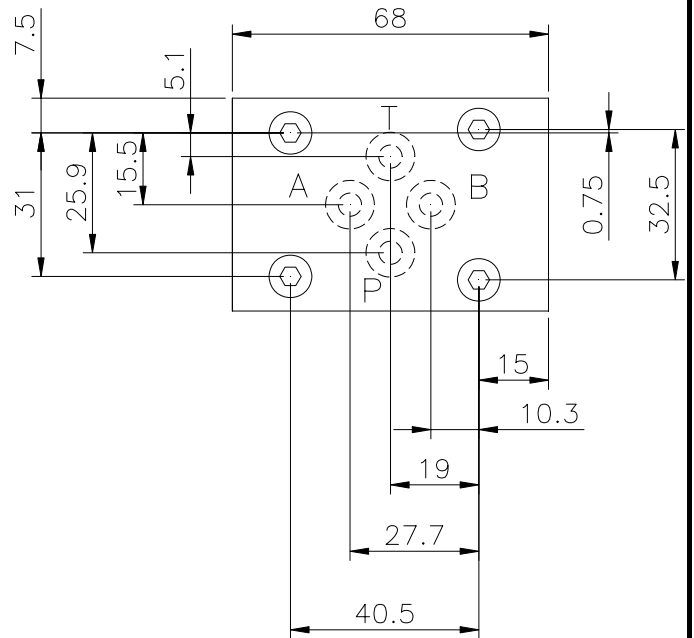
安装面尺寸:
